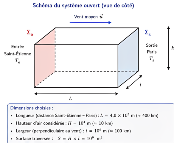
FIGURE 1 – Système ouvert en convection
